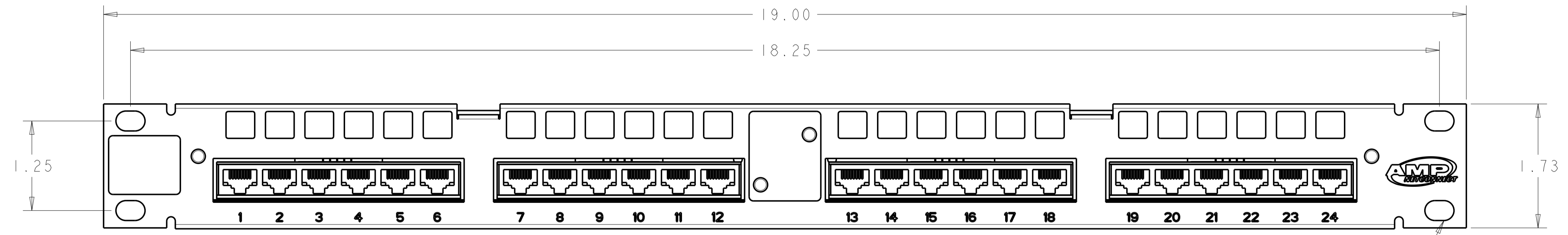
SCALE 1:1 -1 NON-AMPTRAC
