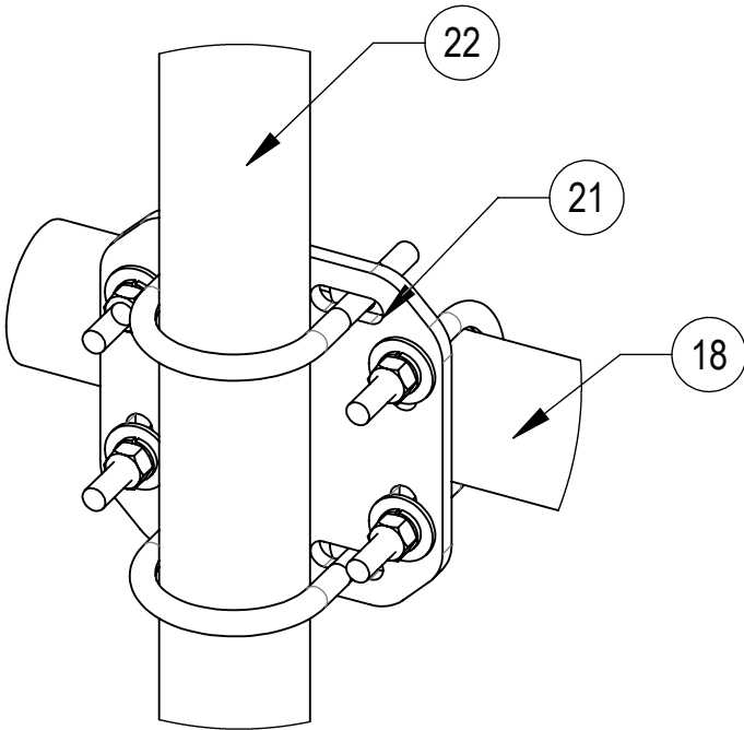
DETAIL Y SCALE 1 : 4
